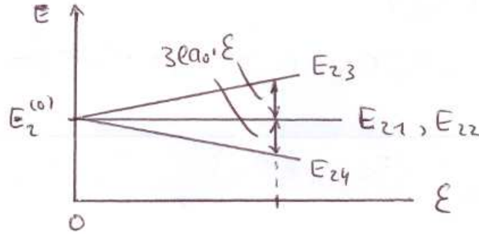
Abbildung 7.2: Linearer Stark-Effekt des Wasserstoff-Energieniveaus n = 2 .
